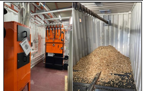
蔵の湯に熱を供給する木質バイオマスボイラ
